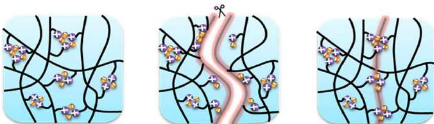
INTERACCIONES IÓNICAS
