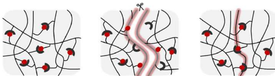
QUÍMICA DIELS-ALDER
